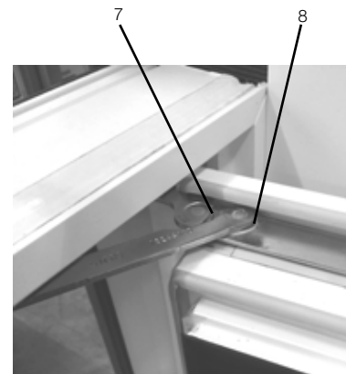
7 8 Schere, Drehlager oben
