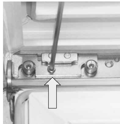
Fixierschraube am Kipplager mit Inbusschlüssel SW4 lösen.
