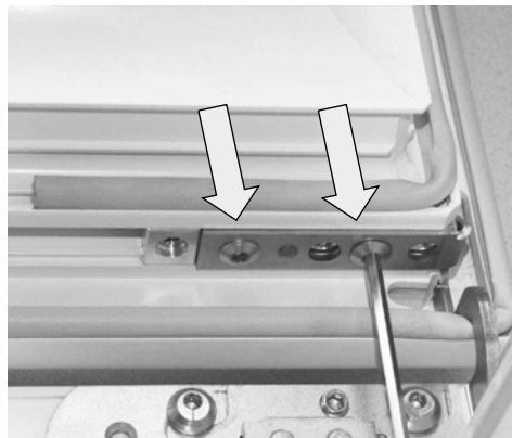
Justierung vertikal Variante b Flügel max. 90° öffnen. Heben und Senken des Flügels abwechselnd mit Inbusschlüssel SW4.
